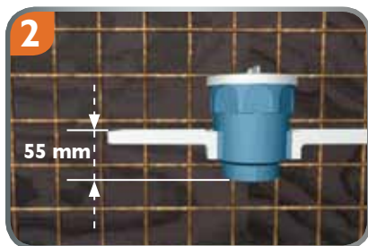
Bei Abstand von 55 mm den Flügel umgedreht aufschieben.
