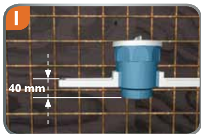
Flügel mit Abstand von 40 mm aufschieben, bei anderem Abstand Flügel drehen.
