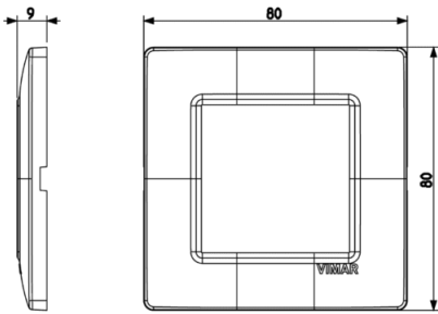
Zeichnung Dimensionen
