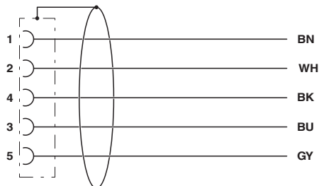
Schaltplan
