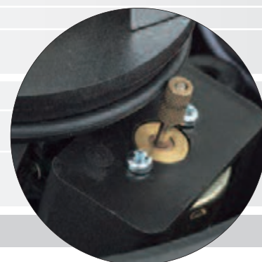
Verschleißarmer Reibradantrieb
