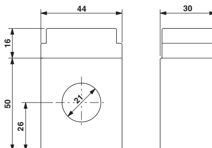
Maßzeichnung
